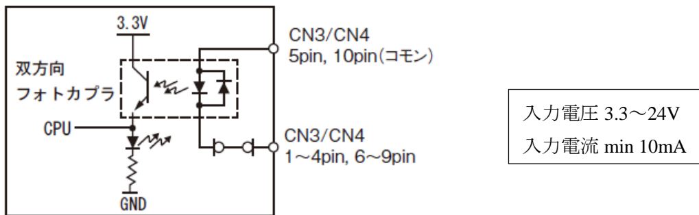
パラレル IO 入力インターフェース (プラスコモン/マイナスコモン共通)
