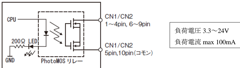
パラレル IO 出力インターフェース (Sink/Source)
